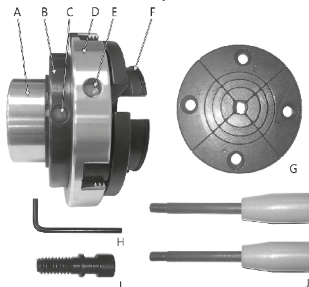
A – хвостовик, B – корпус, C – отверстие для ключа, D – фланец, F – кулачки, G – комплект дополнительных кулачков, H – ключ шестигранный, I – вставка винтовая, J – ключи
